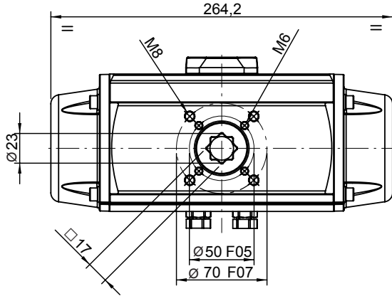
VISTA: DETALLE EJE VIEW: SHAFT DETAIL
