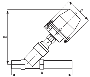
Dimension / Ölçüler
